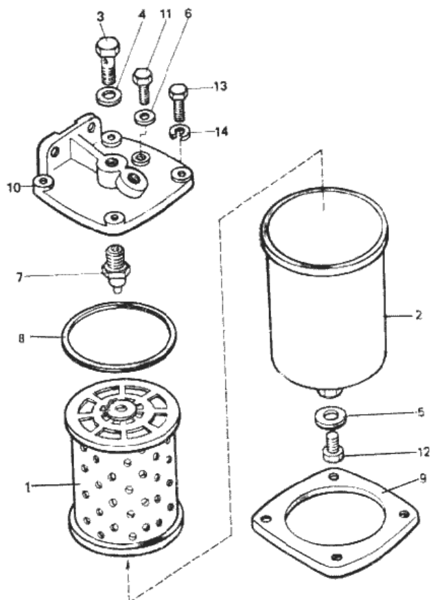
Рис. 25. Фильтр топливный тонкой очистки А65-01.000
